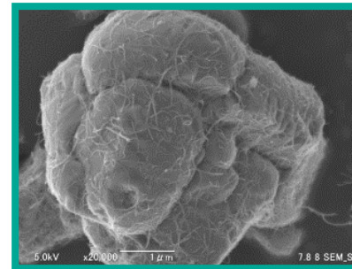
活物質表面に均一に吸着したCNT 正極用導電助剤「CNT分散体」
